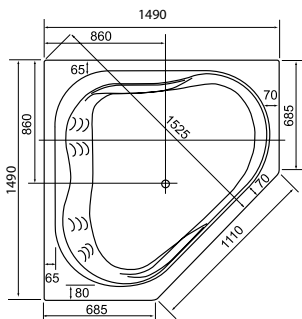
positano - 1490 x 1490 x 540mm
