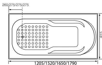
modena - 1205 x 815 x 425mm & 1520 x 815 x 445mm 1650 x 815 x 510mm & 1790 x 815 x 510mm
