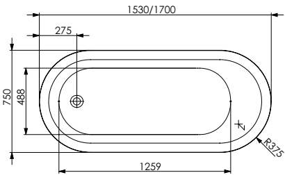
uno - 1530 x 750 x 480mm 1700 x 750 x 490mm
