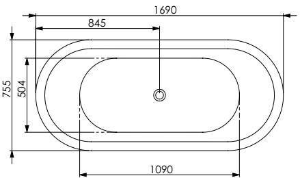
lido - 1690 x 755 x 476mm
