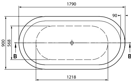
mintori - 1790 x 900 x 595mm(min) - 630mm(max)
