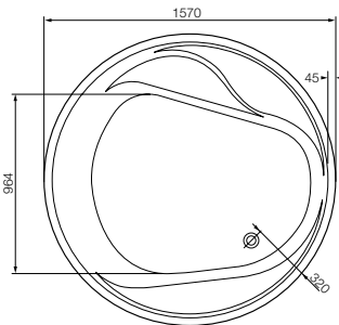
orion - 1570 x 575mm(min) 605mm(max)
