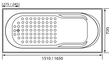
bambino - 1510 x 720 x 410mm 1650 x 720 x 410mm
